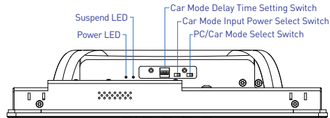
Right I/O
