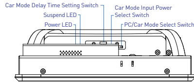
Right I/O
