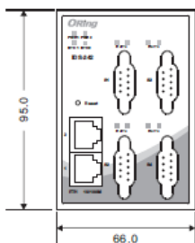
IDS-342
